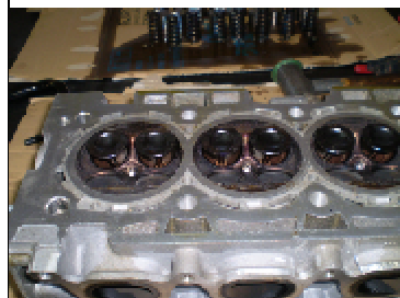
タイミングベルトのトラブルによりシリンダーヘッドのオーバーホール
