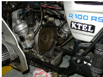
クラッチ オーバーホール
